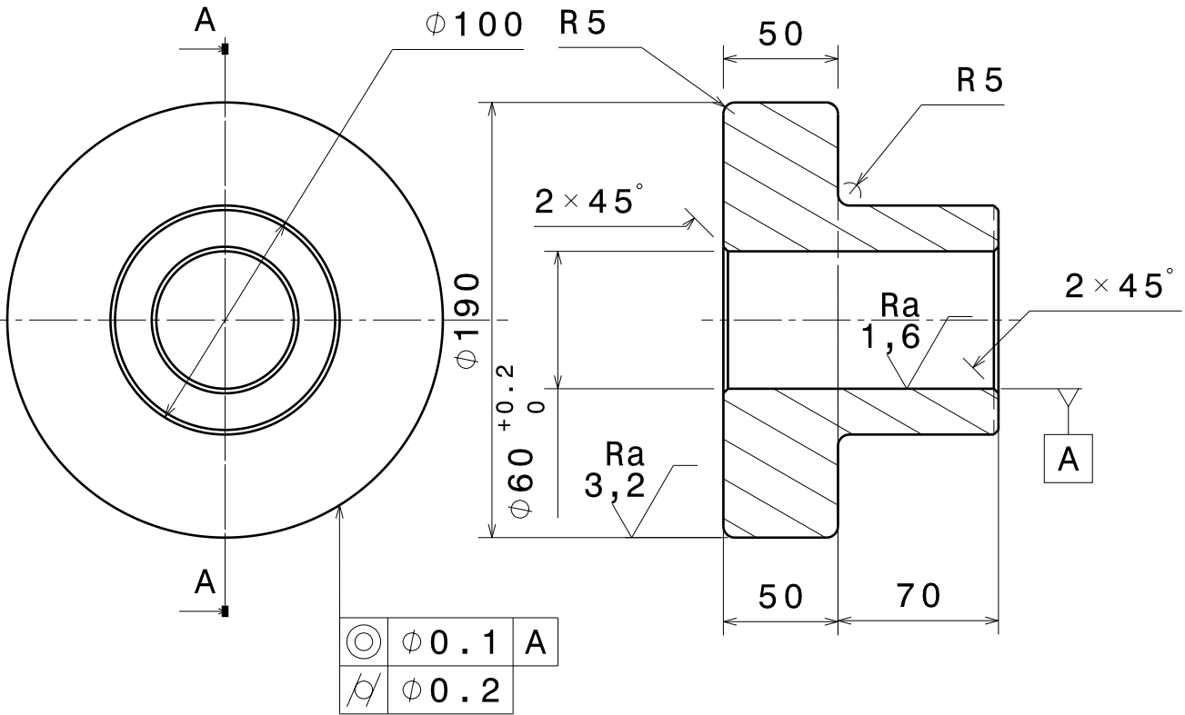
Vue de droite Echelle : 1:3
